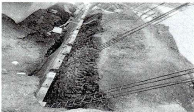
Foto 3: Reparación de muro perimetral de block con tubo hg y malla galvanizada, (soleras intermedias, cimiento de corrido, soleras de humedad, hiladas de block, tubos y columnas).
