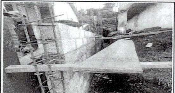
Foto 2: Reparación de muro perimetral de block con tubo hg y malla galvanizada, (soleras intermedias, cimiento de corrido, soleras de humedad, hiladas de block, tubos y columnas).
