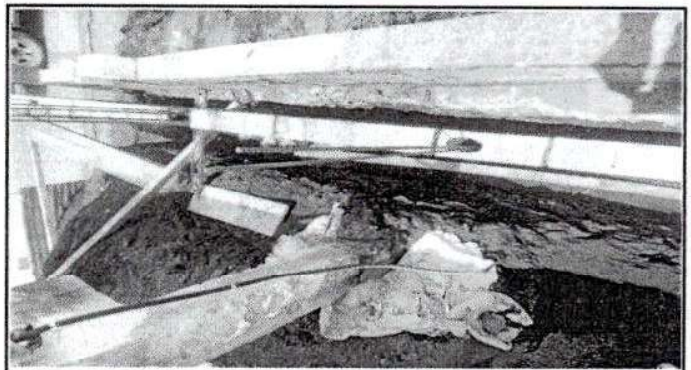
Foto 4: Reparación de muro perimetral de block con tubo hg y malla galvanizada, (soleras intermedias, cimiento de corrido, soleras de humedad, hiladas de block, tubos y columnas).
